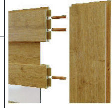
Pevné lepené kolíkové spoje s perodrážkou
