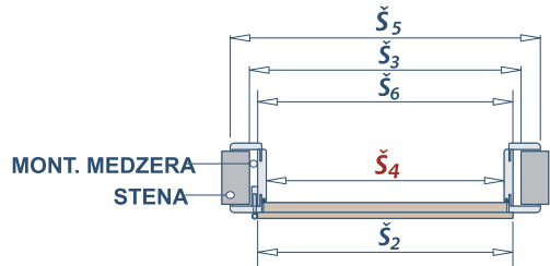
HORIZONTÁLNY REZ
