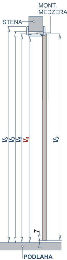
ZVISLÝ REZ
